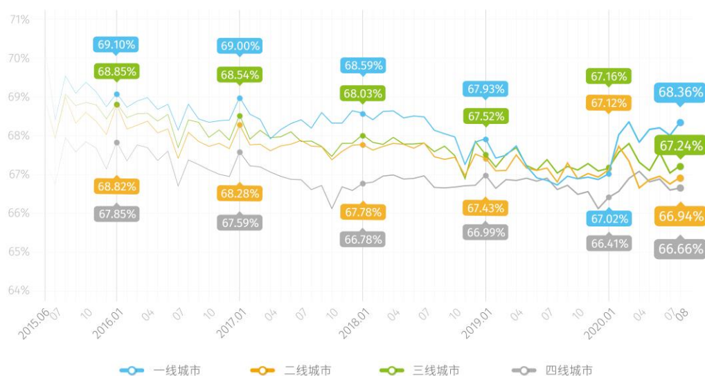
图9-2:不同城市岗位创新性
