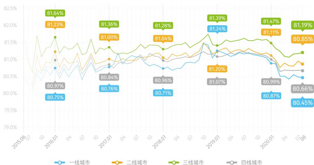
图9-1:不同城市岗位合作性
