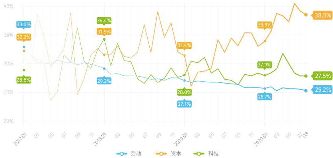
图2:NEI一级指标
