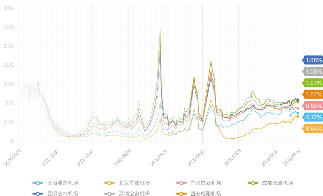
图7:各大机场客流量同比变化
