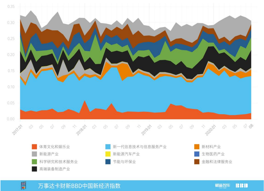
图4:分行业新经济指数
