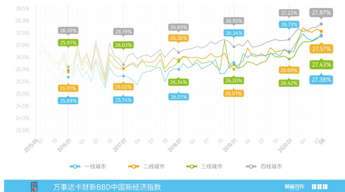
图9-3:不同城市岗位自动化程度
