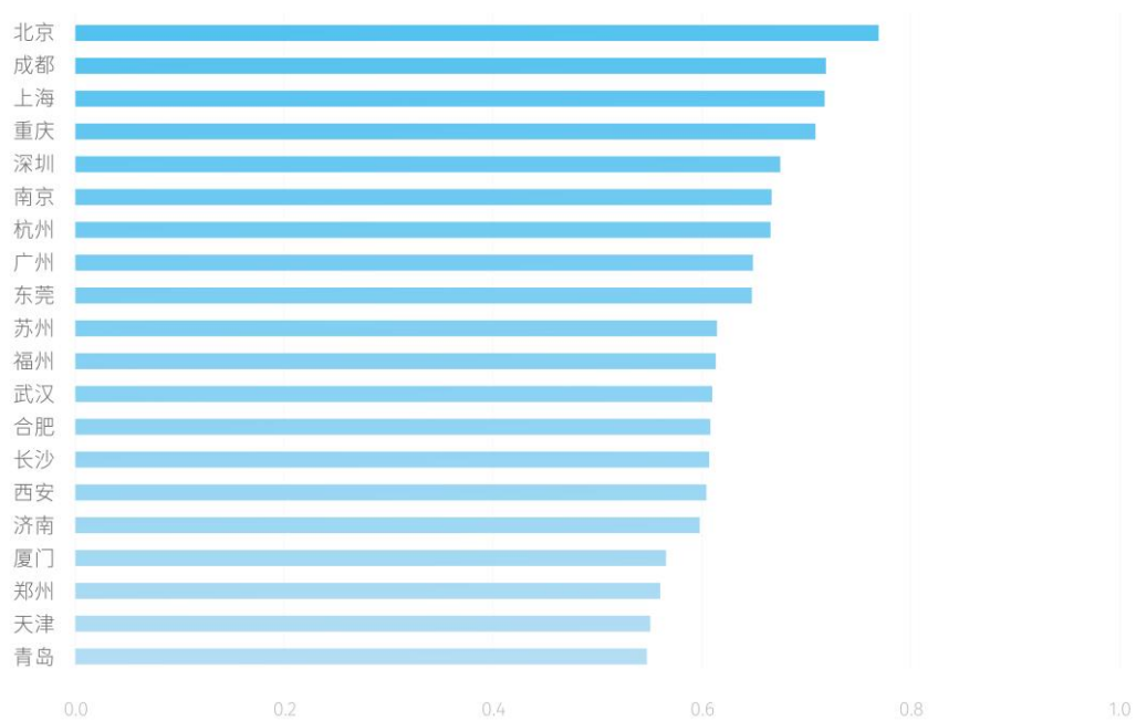
图12:综合成本调整后的总量排名前20名
