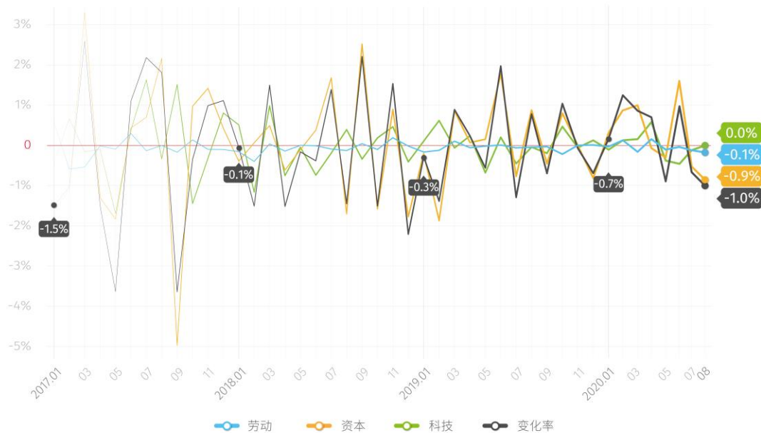
图3:一级指标对各月NEI变化的贡献
